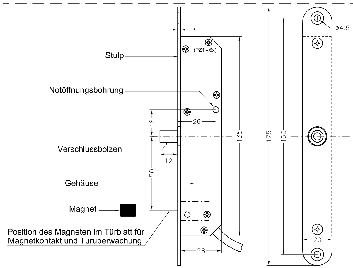
Abbildung 2-2 - Einbaumaße Sperrelement
