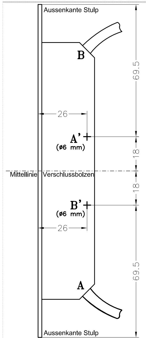
Abbildung 5-1 - Bohrschablone Notöffnung Bohrung (ø6 mm) je nach Position der Kabeleinführung (A) oder (B) an Punkt A' oder B' vornehmen
