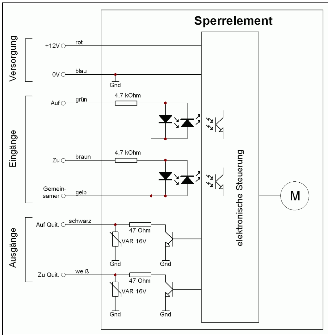
Abbildung 2-3 - Anschlussplan
