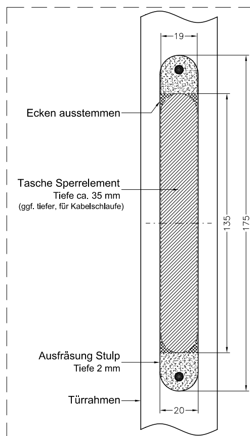
Abbildung 2-1 - Montage Sperrelement
