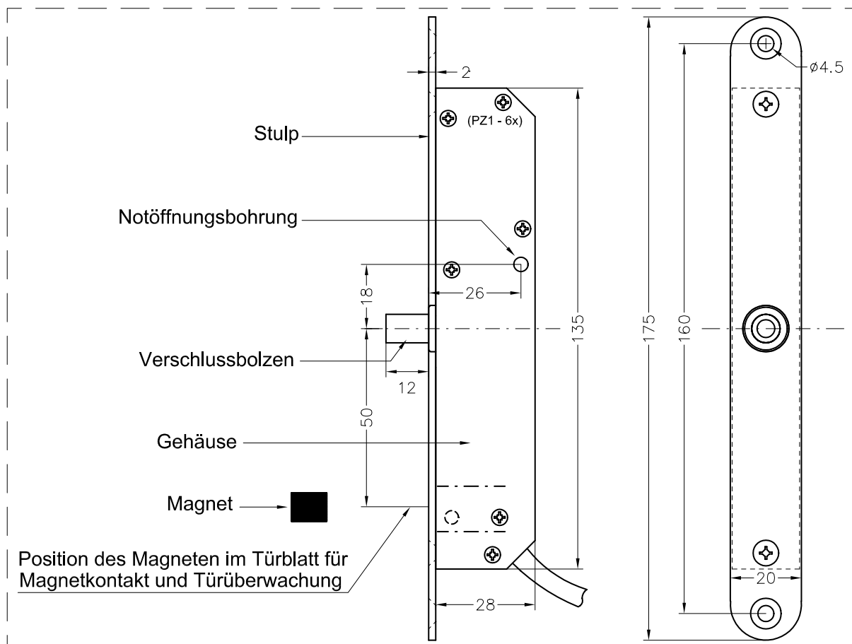
Abbildung 2-2 - Einbaumaße Sperrelement
