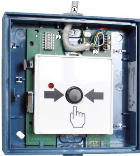
Zugentlastung Anschlussleitung
