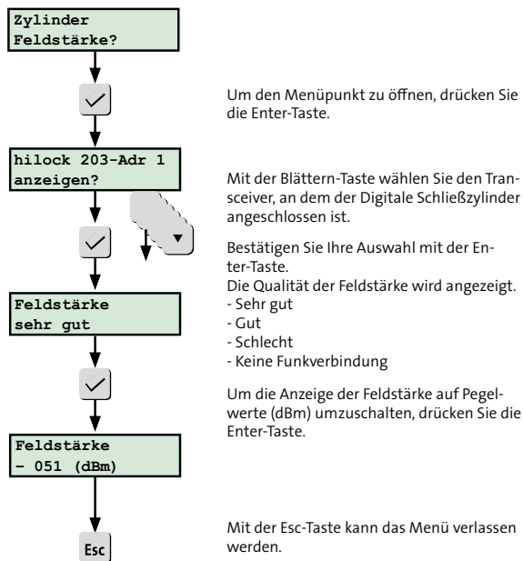
Abb.: Menü Zylinder Feldstärke
