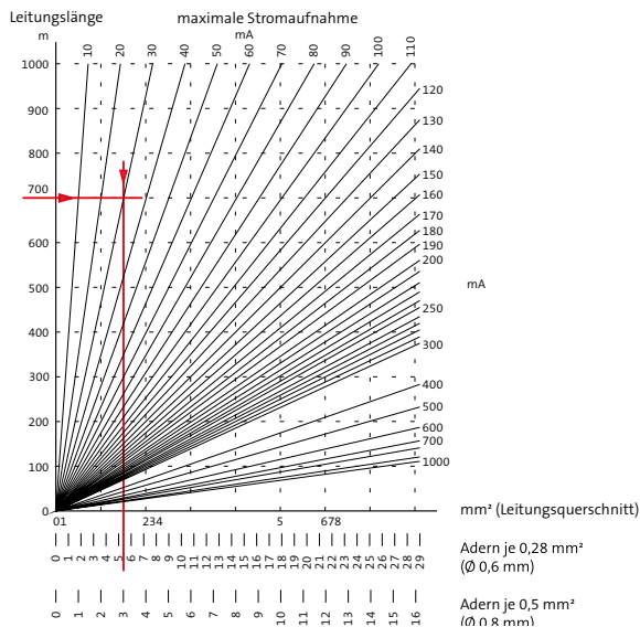
Diagramm zur Ermittlung der Adernanzahl des BUS-1
