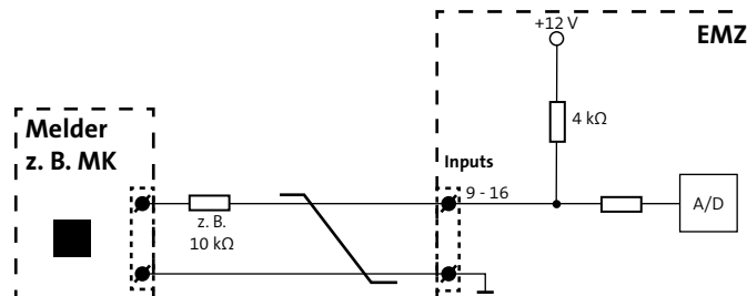
Anschlusschema Inputs 9-16
