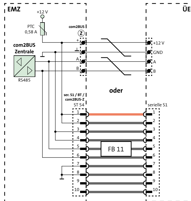
Anschlussschema Schnittstelle ser. S1 / BT / com2BUS-Z
