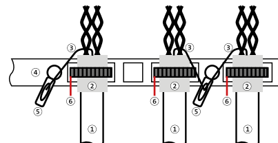
Anschluss Schirmung mit Lötösen
