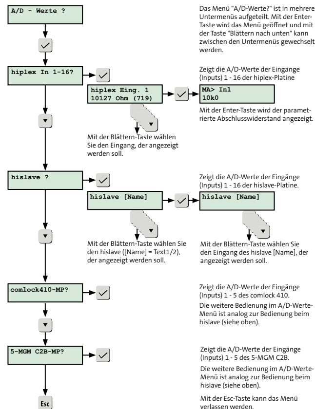
Abb.: Menü A/D-Werte
