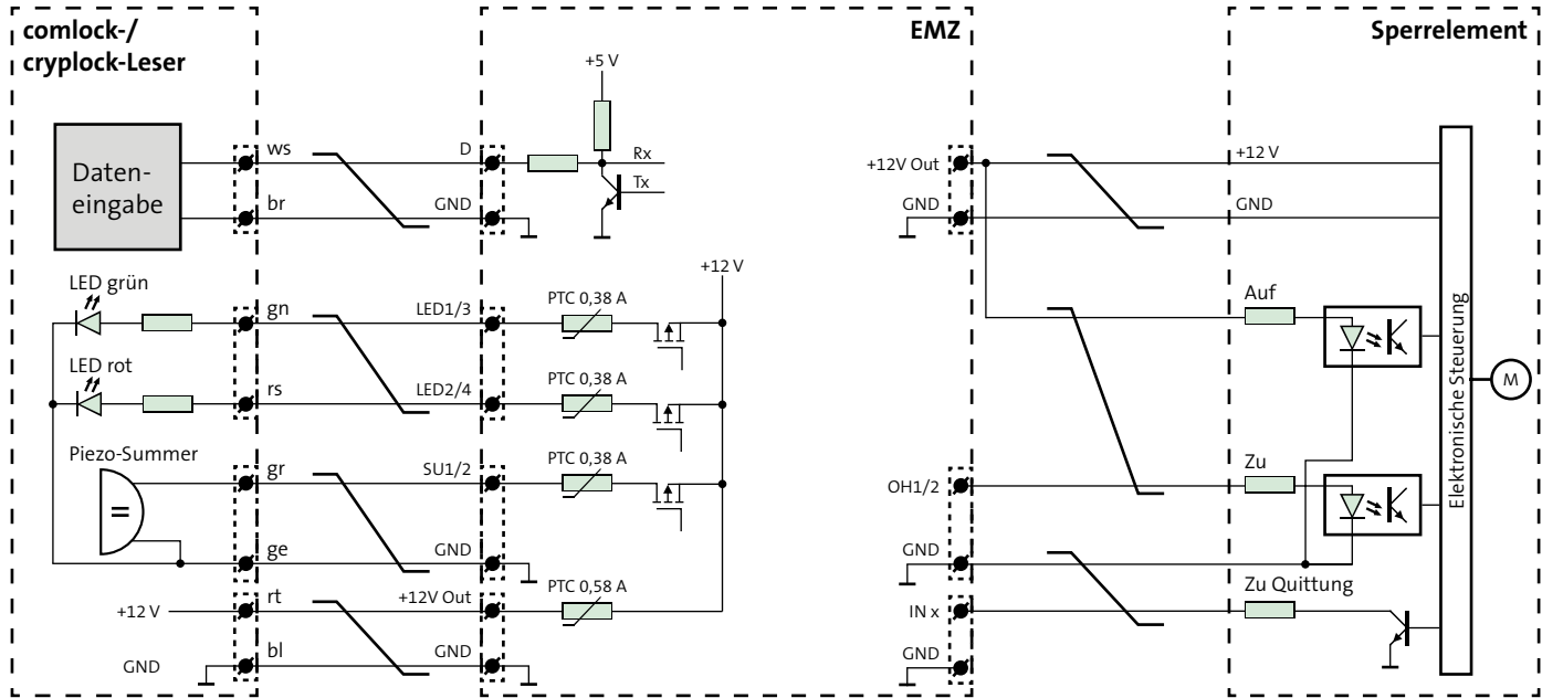
Anschlussschema comlock-/cryptlock-Leser (Reader 1/2)
