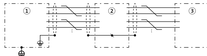
Abb.: Schirmung mehrerer Geräte mit Kunststoffgehäuse
