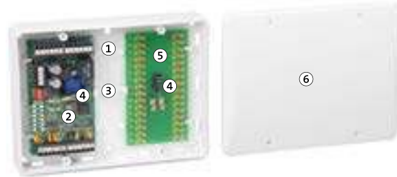
Mechanischer Aufbau Türmodul comlock 410 aP-Montage mit Lötverteiler im Gehäusetyp K30
