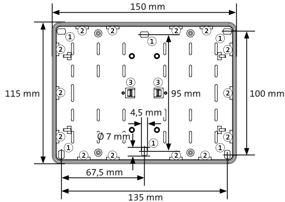
Maßzeichnung Gehäusetyp K30
