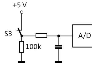
Schema Sabotagekontakt
