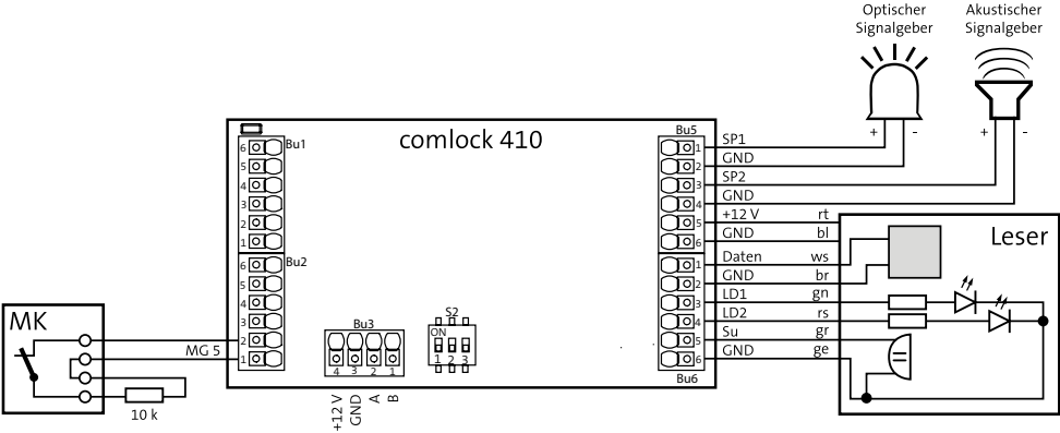
Anschaftbeispiel Betriebsart Tagalarm mit comlock-/cryplock-Leser
