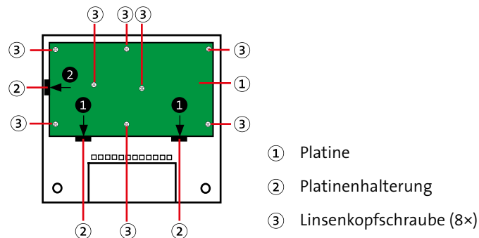
Montage Platine
