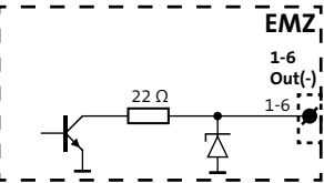
Anschlussschema Transistorausgänge 1-6 Out (-)
