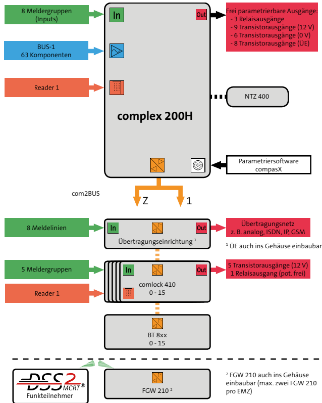
Funktionsschema EMZ
