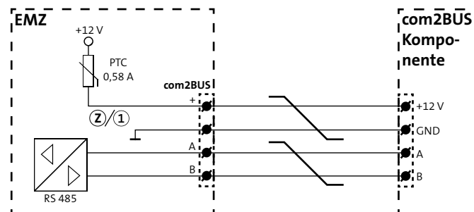
Anschlussschema com2BUS
