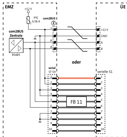
Anschlussschema Schnittstelle serial
