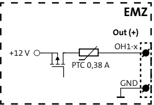
Anschlussschema Spulenausgänge (OH1-2)
