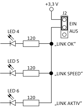
J2 zur Abschaltung von LED 4–6
