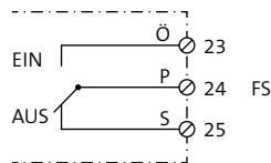
Ausgang „FS“
