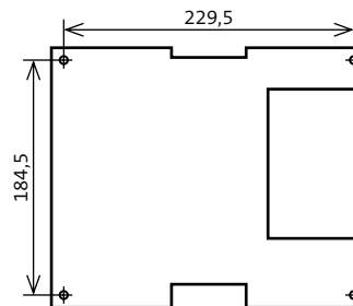
Maßzeichnung Gehäusetyp S3
