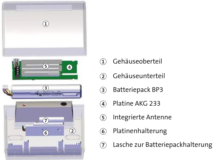
Aufbau Akustischer Glasbruchmelder Funk AKG 233
