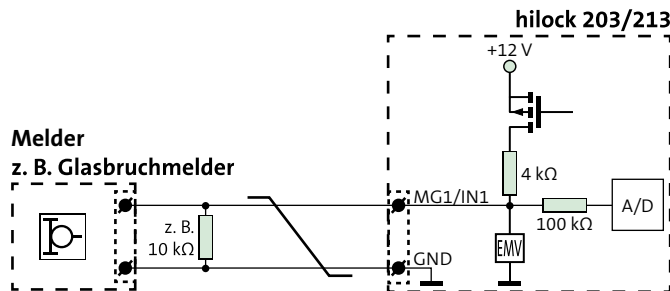
Anschlusschema MG1/IN1
