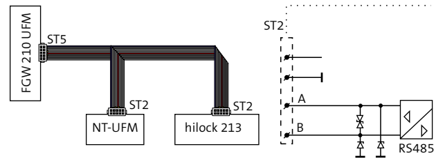
Flachbandleitung für die com2BUS-Verbindung
