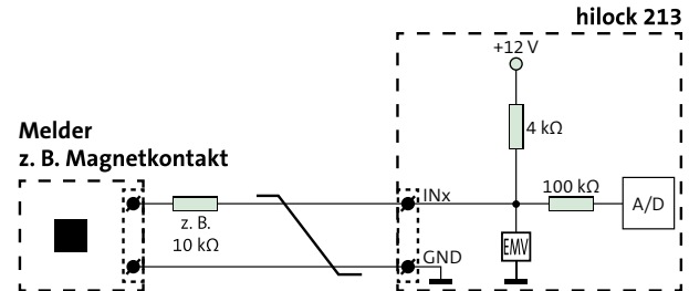
Anschlussschema IN2-3
