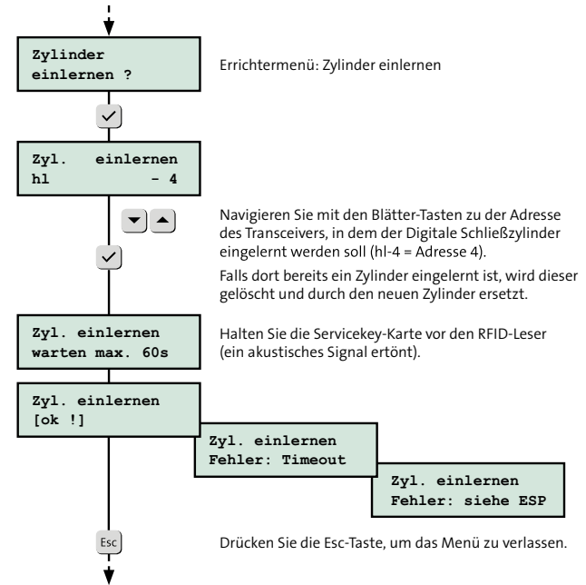
Digitaler Schließzylinder einlernen (EMZ complex 200H/400H)
