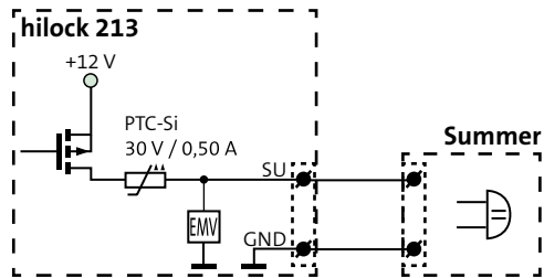
Anschlusschema SU
