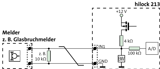
Anschlussschema IN1
