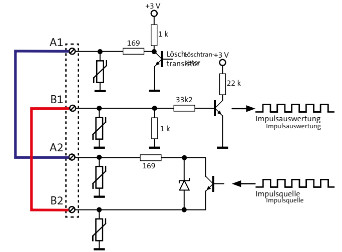
Blockschaltbild multifunktionaler Eingang in Ruhe
