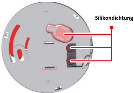
Abb. 2 Sockel
