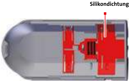
Abb. 2 Gehäuseunterteil
