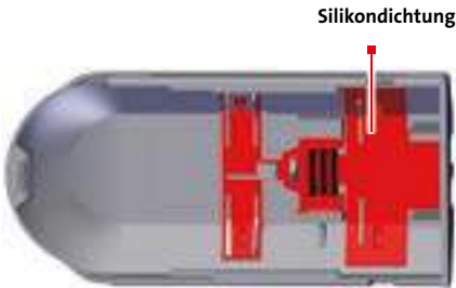
Abb. 2 Gehäuseunterteil
