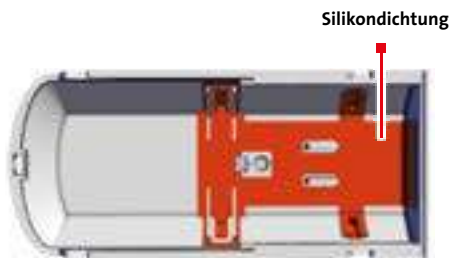
Abb. 2 Gehäuseunterteil
