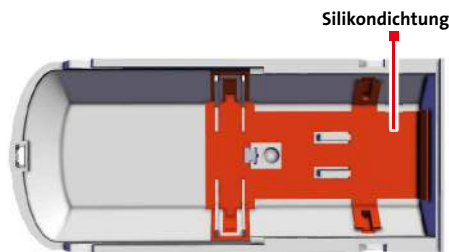
Abb. 2 Gehäuseunterteil
