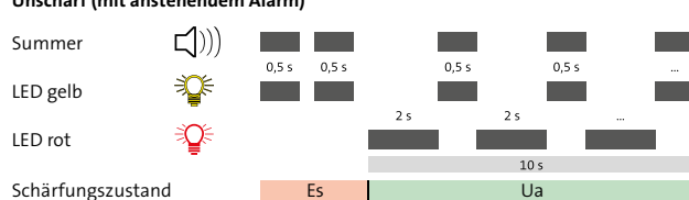
Zweistufige Unscharfschaltung (Tastaturcode und Transponder) am cryplock-Leser
