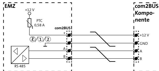
Anschlusschema com2BUS
