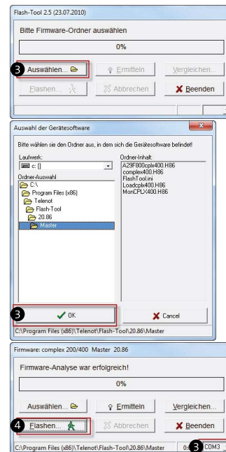
Flash-Tool-Software
