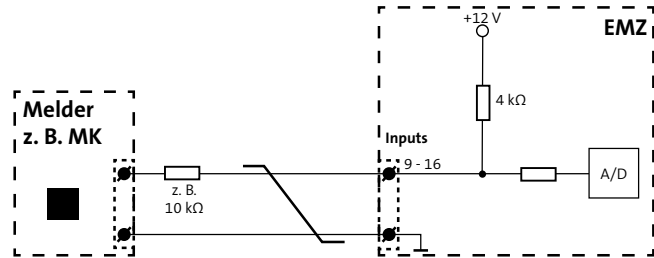
Anschlussschema Inputs 9-16
