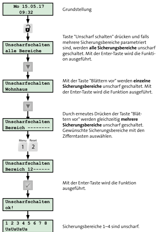
Unscharf schalten am BT 820
