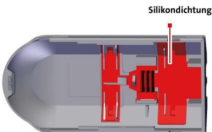
Abb. 2 Gehäuseunterteil
