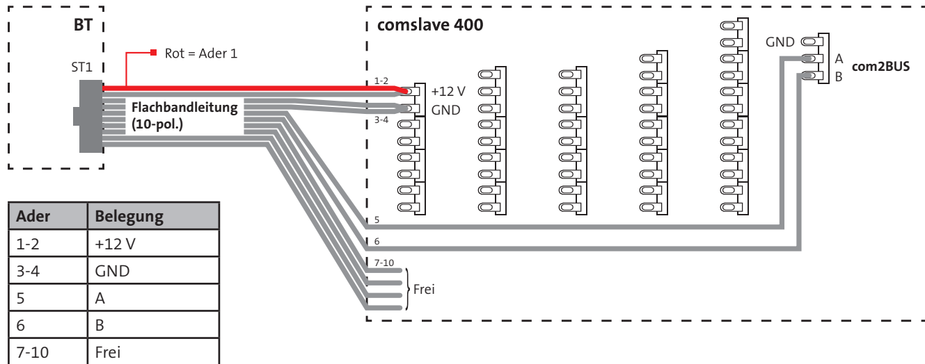
Anschlussbelegung
